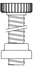
YBφ302"手締めナット付 (2"三角PK付)
