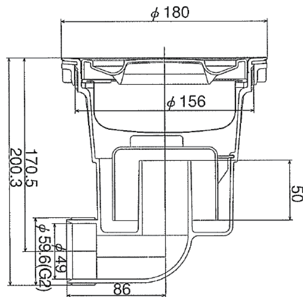
排水トラップ寸法図
