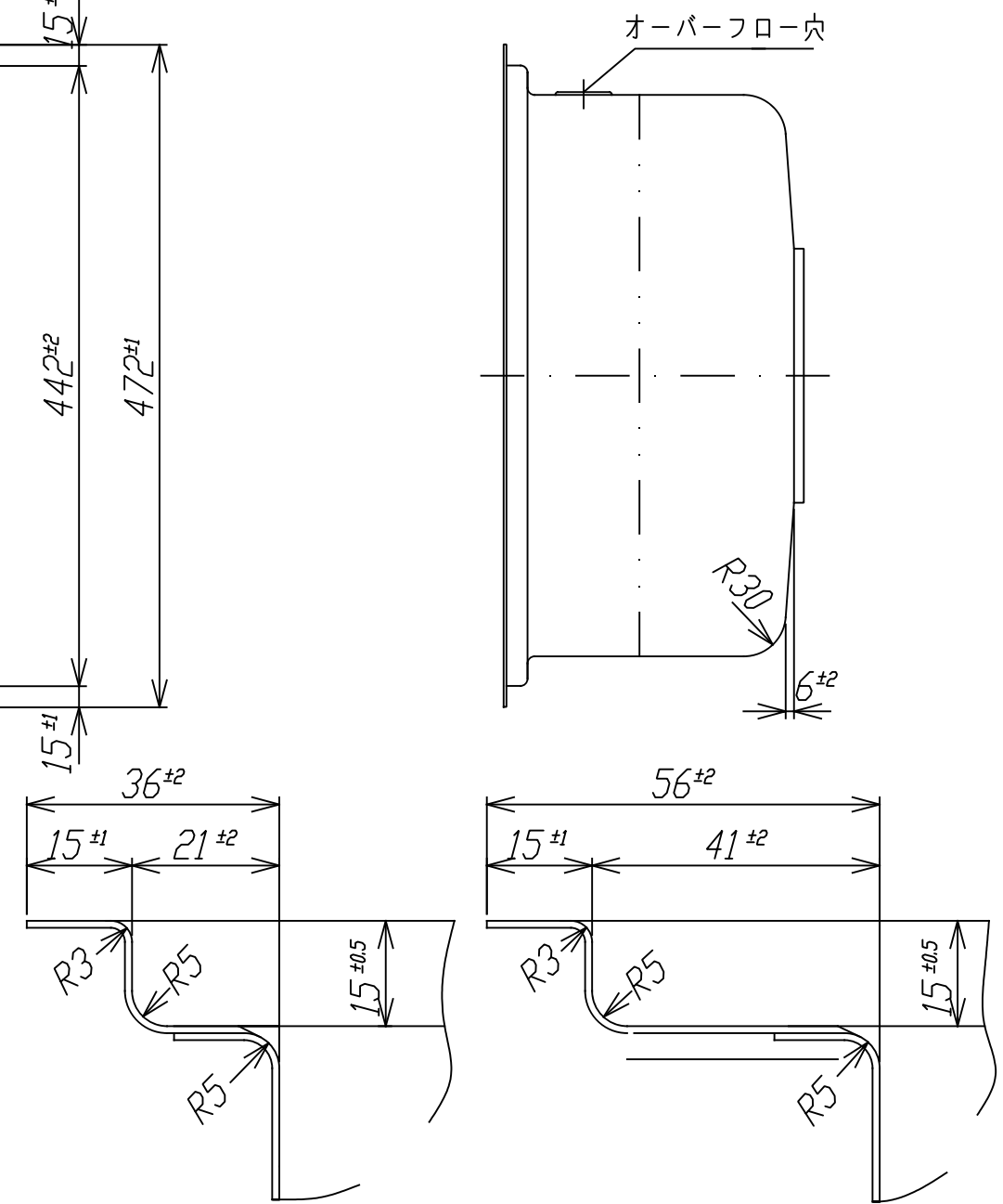
A-A'断面 S=1/1 B-B'断面 S=1/1
