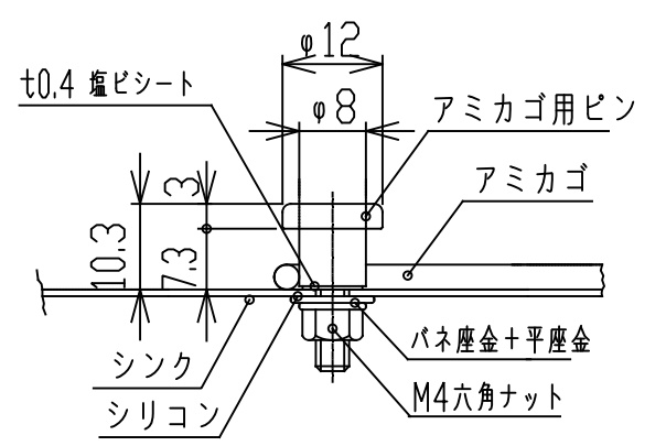
アミカゴ用ピン取付詳細 S = 1 / 1
