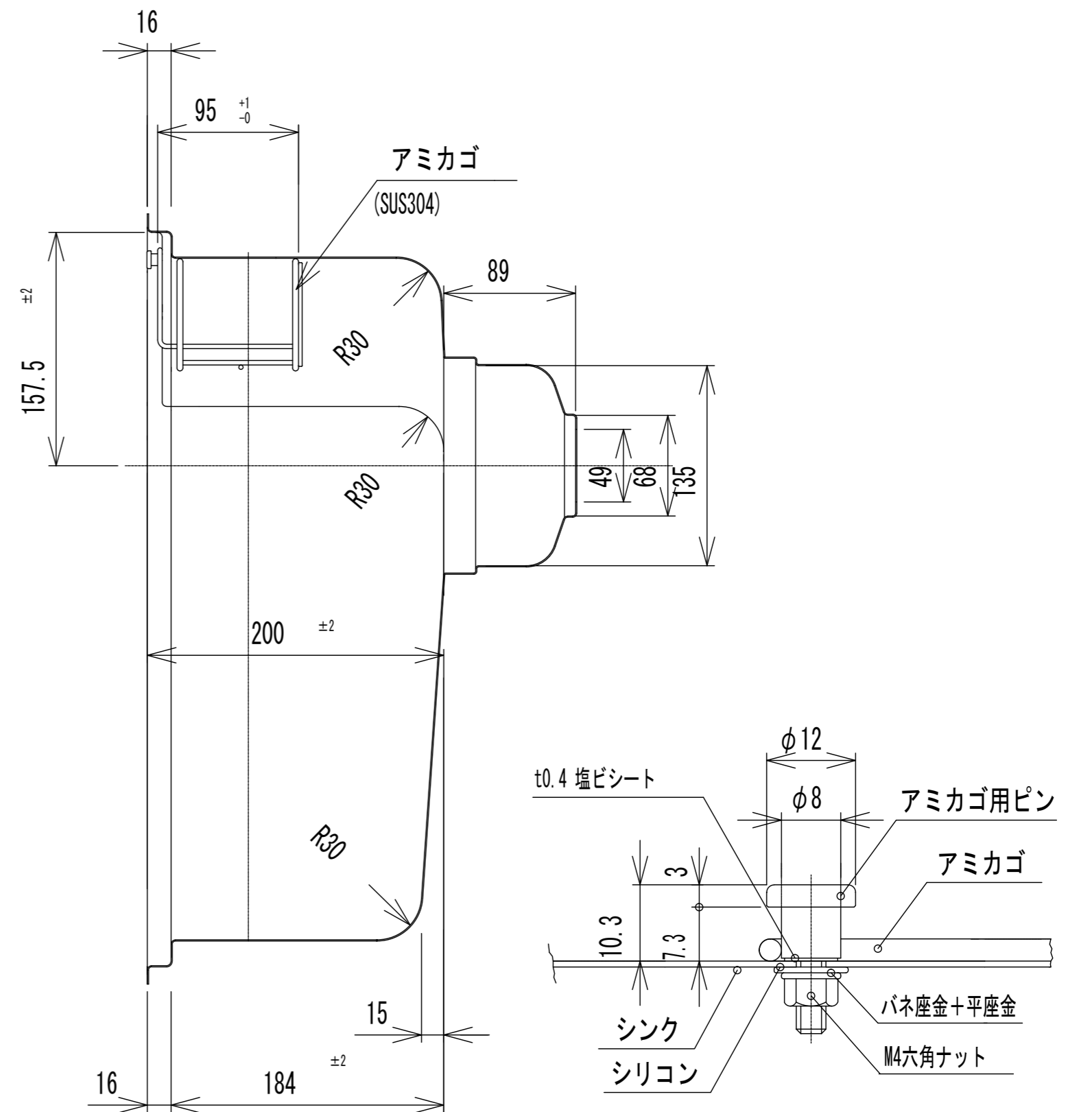
アミカゴ用ピン取付詳細 S=1/1
