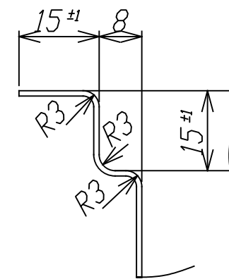
A-A'断面 S=1/1
