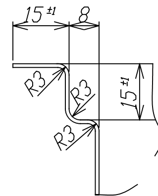
B-B'断面 S=1/1
