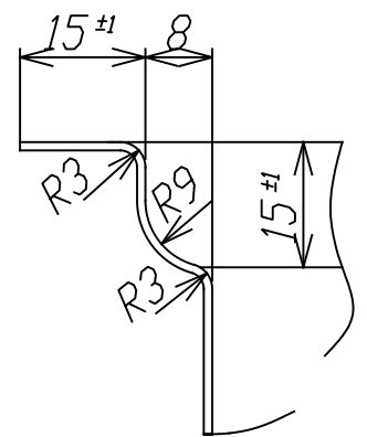
C-C'断面 S=1/1
