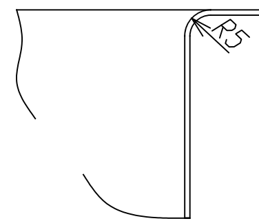
A-A'断面 S=1/1
