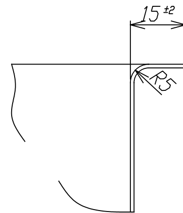
A-A'断面 S=1/1
