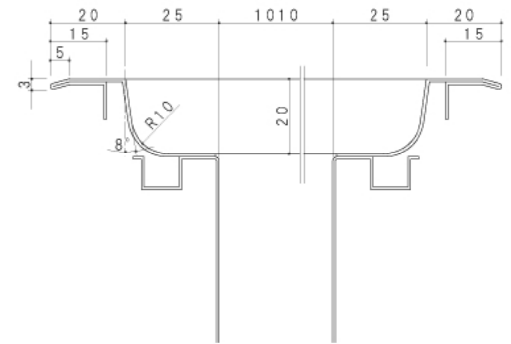
AA断面 (1/1)
