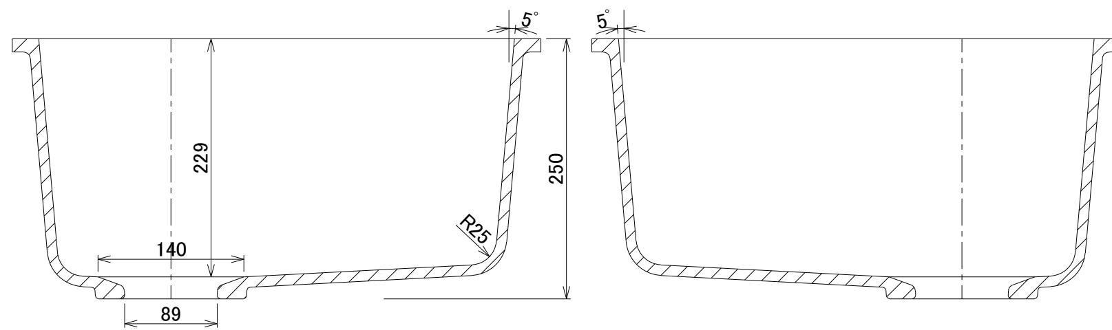
A-A 断面図
