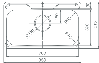
COMO-V8 アンダータイプ COMO-V8-○ オーバータイプ ボール深さ:205 水栓孔径:36φ 排水孔径:159φ 生地:18-8ステンレス 裏面:防震材 (イシバシテクノ製) 排水トラップ:φ180用
