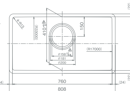
COMO-S15R アンダータイプ ボール深さ:190 排水孔径:158φ 生地:18-8ステンレス 裏面:防震材 (トヨウラ製) 排水トラップ:φ000用
