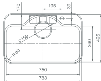
COMO-FCM アンダータイプ ボール深さ:200 水栓孔径:36φ 排水孔径:159φ 生地:18-8ステンレス 裏面:防震材 (シゲル製) 洗剤カゴ付 排水トラップ:φ180用
