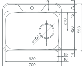
COMO-G6(R) アンダータイプ COMO-G6-○(R) オーバータイプ ボール深さ:203 水栓孔径:36φ 排水孔径:160φ 生地:18-8ステンレス 裏面:防震材 (イシバシテクノ製) 排水トラップ:φ180用
