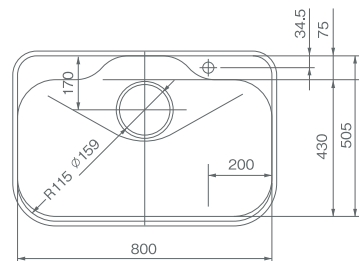
COMO-C8 アンダータイプ ボール深さ:190 水栓孔径:36φ 排水孔径:159φ 生地:18-8ステンレス 裏面:防震材 (トヨウラ製) 洗剤カゴ付 排水トラップ:φ180用
