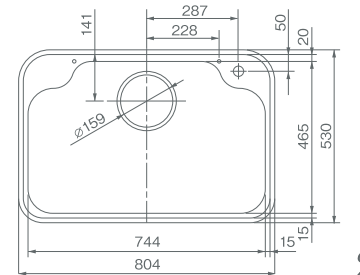
COMO-IB アンダータイプ ボール深さ:181 水栓孔径:36φ 排水孔径:159φ 生地:18-8ステンレス 裏面:防震材 (シゲル製) 洗剤カゴ付 排水トラップ:φ180用
