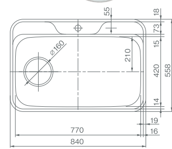
COMO-G8(L) アンダータイプ COMO-G8-○(L) オーバータイプ ボール深さ:203 水栓孔径:36φ 排水孔径:160φ 生地:18-8ステンレス 裏面:防震材 (イシバシテクノ製) 排水トラップ:φ180用
