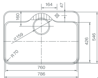
COMO-GB アンダータイプ ボール深さ:200 水栓孔径:36φ 排水孔径:159φ 生地:18-8ステンレス 裏面:防震材 (シゲル製) 洗剤カゴ付 排水トラップ:φ180用
