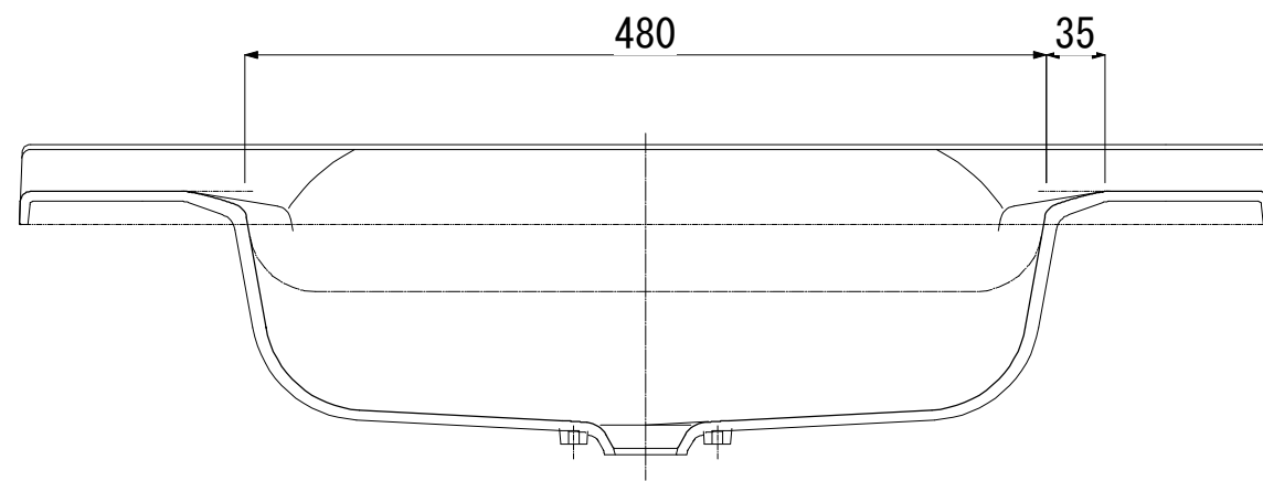
断面図 B - B
