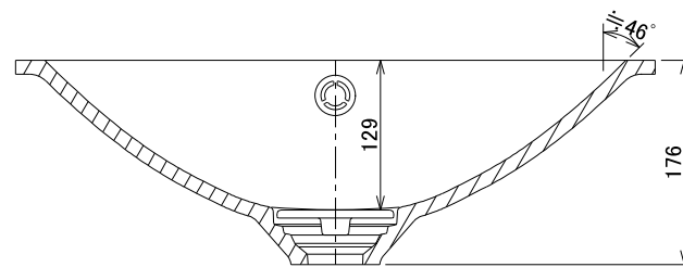
A-A 断面図
