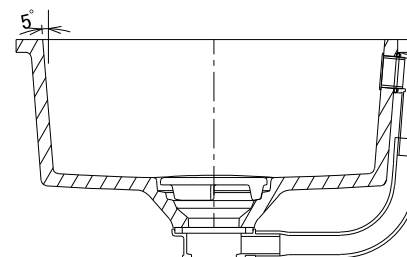
B-B 断面図
