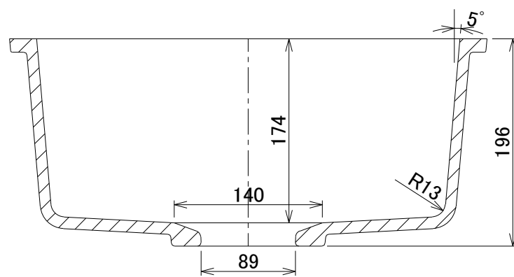
A-A 断面図
