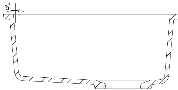
B-B 断面図
