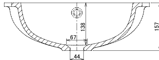
A-A 断面図
